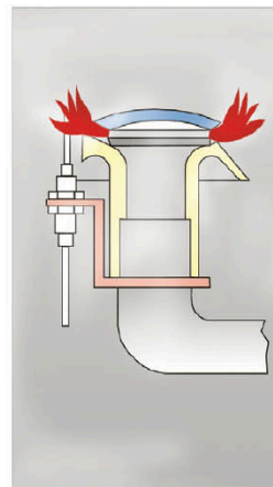
Sl.11. Plavičasti plamen bez žutih vrhova i bez dima znak je da je usklađen omjer plina i zraka potreban za normalno i potpuno sagorijevanje plina. Plamen na pomoćnom plameniku mora biti dug 35-40 mm. Treba izbjegavati suviše malen plamen jer bi se on mogao ugasi iznenadnim zračnim strujanjem, prelijevanjem hrane ili pogrešno izvedenom instalacijom. Duljina svih plamičaka na plamenicima mora biti izjednačena te moraju gorjeti svjetlo plavim plamenom.
