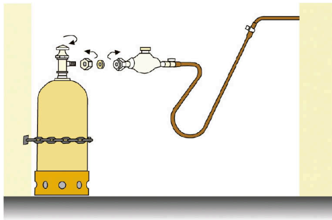
Sl. 8. Plin u bocama Propan-butan plin u bocama primjenjiv je tamo gdje je potrebna fleksibilna i lako prenosiva energija, a jednostavno se i sigurno distribuira do najudaljenijih mjesta.
