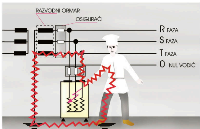
Sl. 5. Indirektni napon dodira nastaje kada metalno kućište koje inače nije pod naponom- npr. bojler, električni štednjak i sl. uslijed proboja izolacije i sl. dođe pod napon (napon greške). Što je manji otpor prolasku električne struje kroz tijelo čovjeka i veći napon na kućištu, kroz čovjeka prolazi jača struja prema poznatom izrazu I = U/R . ( I jakost struje u amperima, U je napon u voltima te R otpor u omima). Važno je i vrijeme trajanje udara. Smrt može nastupiti kada je napon izmjenične struje veći od 50 V (u normalnim uvjetima), ali i kod manjeg napona u ekstremnoj vlažnosti i dodira s metalom po većoj površini tijela.
