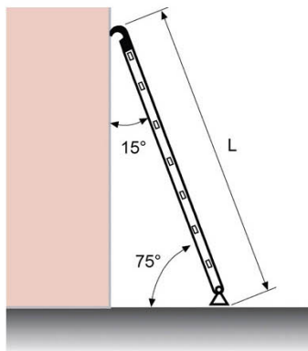
Sl. 23. Jednokrake ljestve se postavljaju pod kutom od 75° prema podu, odnosno 15° prema zidu. Ljestve se trebaju čvrsto oslanjati s oba kraka na gornji i donji oslonac. Ljestve treba postavljati na ravan i čvrst teren. Ljestve moraju biti ispravne, neoštećene, a prečke pravilno učvršćene i razmaknute. Jednokrake ljestve se koriste za penjanje i sasvim iznimno za obavljanje manjih radova.
