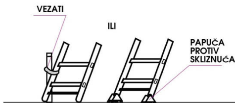
Sl. 22. Donji kraj ljestvi mora se imobilizirati i to vezanjem, učvršćivanjem ili gumenim podmetačima (papučama).
