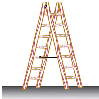
Sl. 25. Dvokrake ljestve služe za penjanje i vršenje radova. Dvokrake ljestve su ispravne samo ako su cijele, prečke usađene, te krakovi učvršćeni međusobno užetom ili lancem. Ljestve moraju biti izrađene prema propisima.
