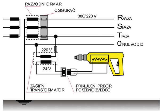
Sl. 6. Ručni električni alat priključen na maleni sigurnosni napon od 24 V izmjenične struje tzv. trošilo klase III.
